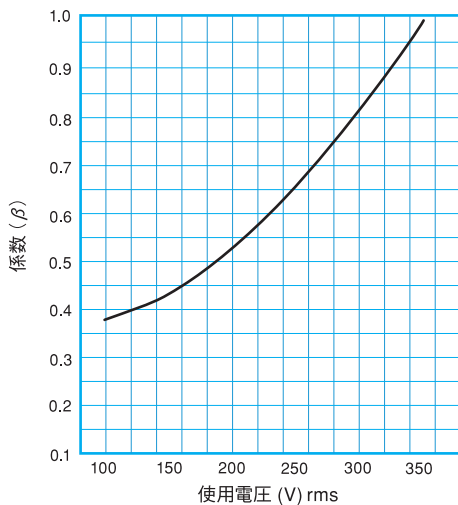
交流使用電圧に対する全遮断 I²t
